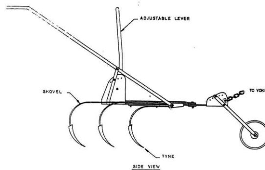
Fig. 18.4 Junior hoe
