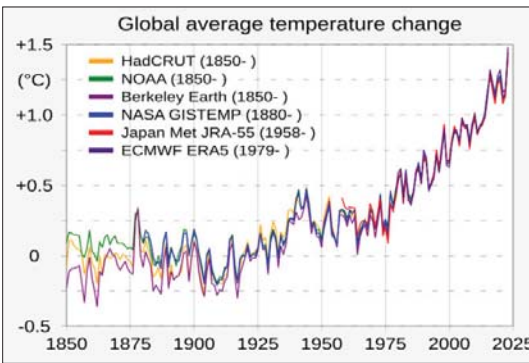
ကမ္ဘာ့ပျမ်းမျှအပူချိန်သည် စက်မှုခေတ်မတိုင်မီ ကာလထက် ပိုမိုမြင့်တက်လာပုံ။
