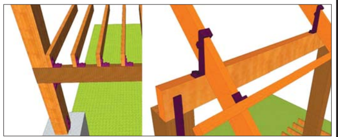
လေပြင်းဒဏ်ကိုခံနိုင်ရန် တိုင်နှင့် ထုပ်တန်းများ၊ ထုပ်နှင့် ခိုင်း၊ ခိုင်းနှင့် မြားတန်း စသည်တို့ကို Brackets များနှင့်လည်း ယခုကဲ့သို့ ချိတ်ဆွဲထားသင့်သည့် ပုံစံငယ်။
