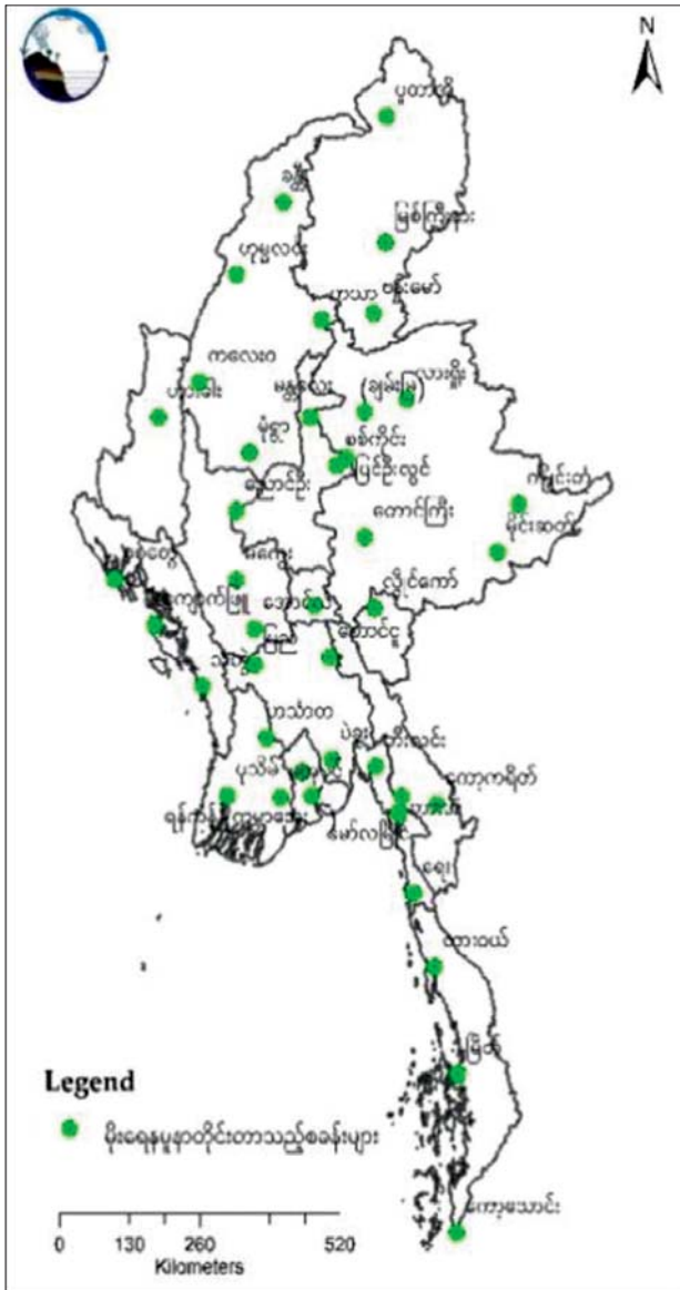
၂၀၂၅ ခုနှစ် ဇူလိုင်လအတွင်း ရွာသွန်းခဲသော မိုးရေဓာတ်တိုင်းတာမှုများ၏ pH တန်ဖိုးများ
