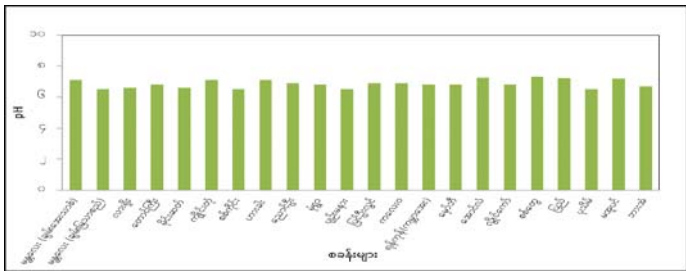
၂၀၂၆ ခုနှစ်၊ မတ်လအတွင်း ရွာသွန်းခဲသော မိုးရေဓာတ်များ၏ pH တန်ဖိုးများ
