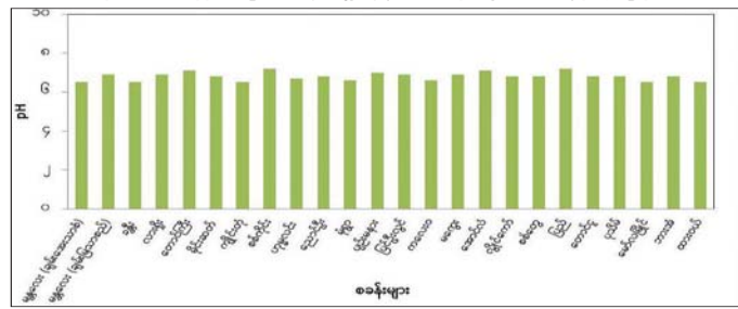
ပုံ (၂)၊ ၂၀၂၆ ခုနှစ်၊ ဧပြီလအတွင်း ရွာသွန်းခဲသော မိုးရေ၏ pH တန်ဖိုးများပြပုံ
